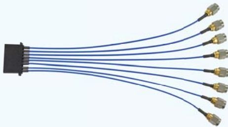
WMA8極 /J WMA8極 /J Assy (08X0636#□□□□)
